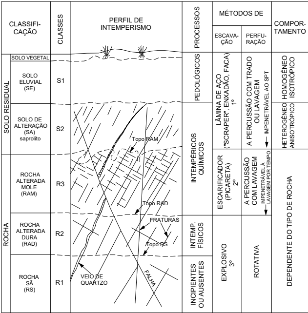
Figura 3 – Perfil de intemperismo em regiões tropicais associado a métodos de perfuração e escavação.
