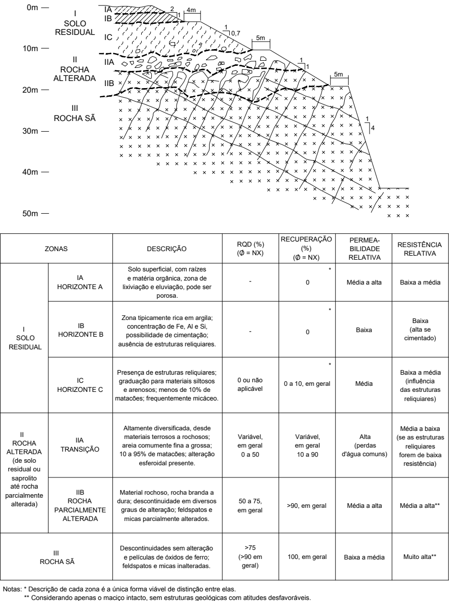
Figura 1 – Perfil de alteração de rochas ígneas e metamórficas, respectivas soluções típicas para taludes de corte e indicação da expectativa de parâmetros geotécnicos.
