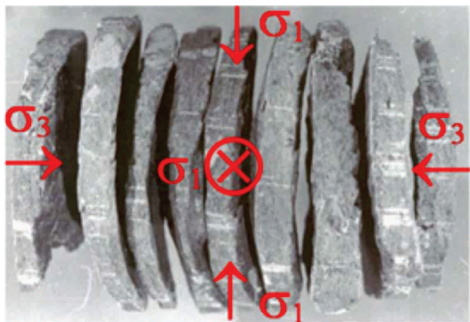
Figura 18c – Disco curvos em forma de prato e as tensões atuantes. Fonte: adaptado de FIGUEIREDO, 2013.
