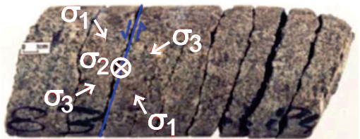
Figura 18d – Discos planares e as tensões atuantes. Fonte: adaptado de FIGUEIREDO, 2013.
