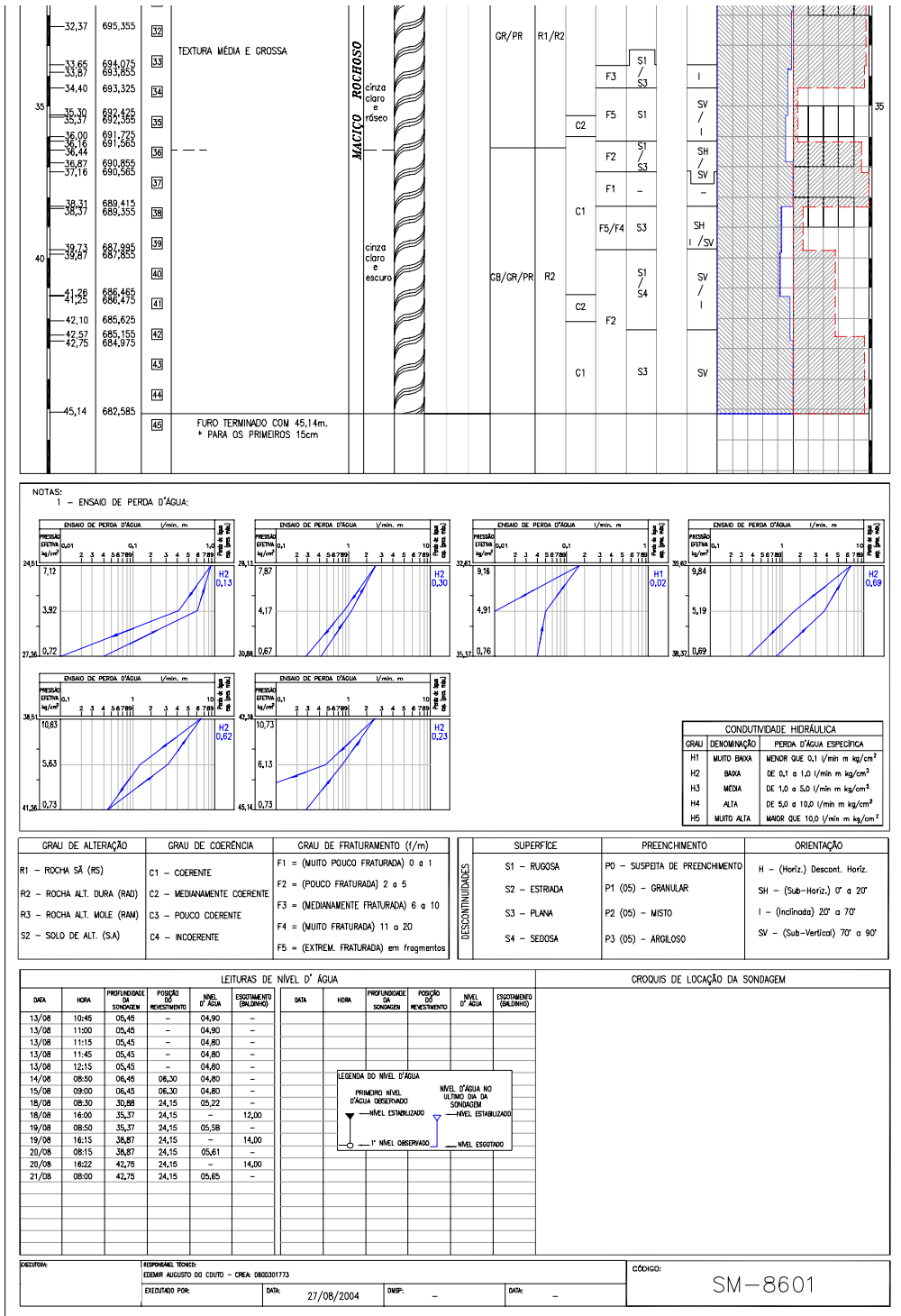
Figura 43 – Exemplo de perfil individual de sondagem mista. Fonte: modificado de Monticeli e Tressoldi (2013).
